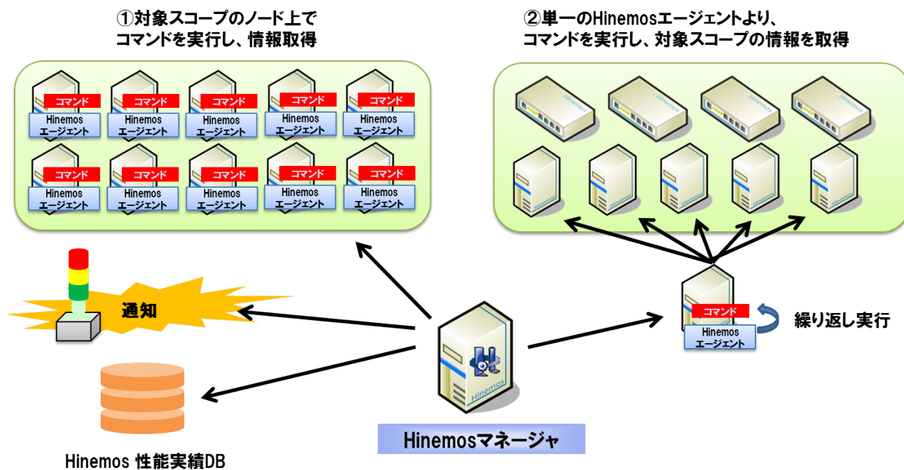
図 7-22 コマンドの実行単位
