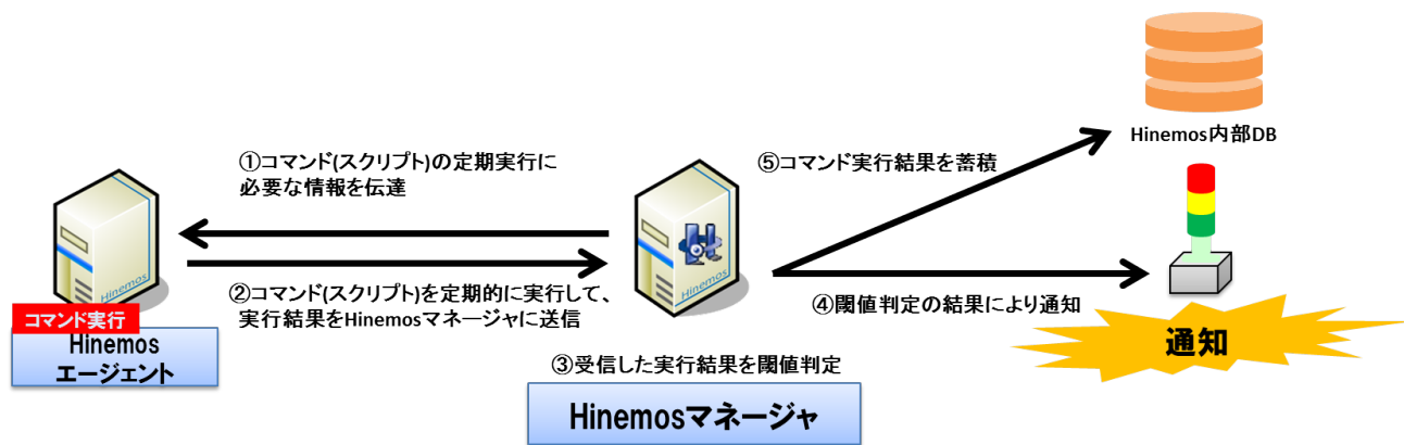
図 7-21 カスタム監視概要
