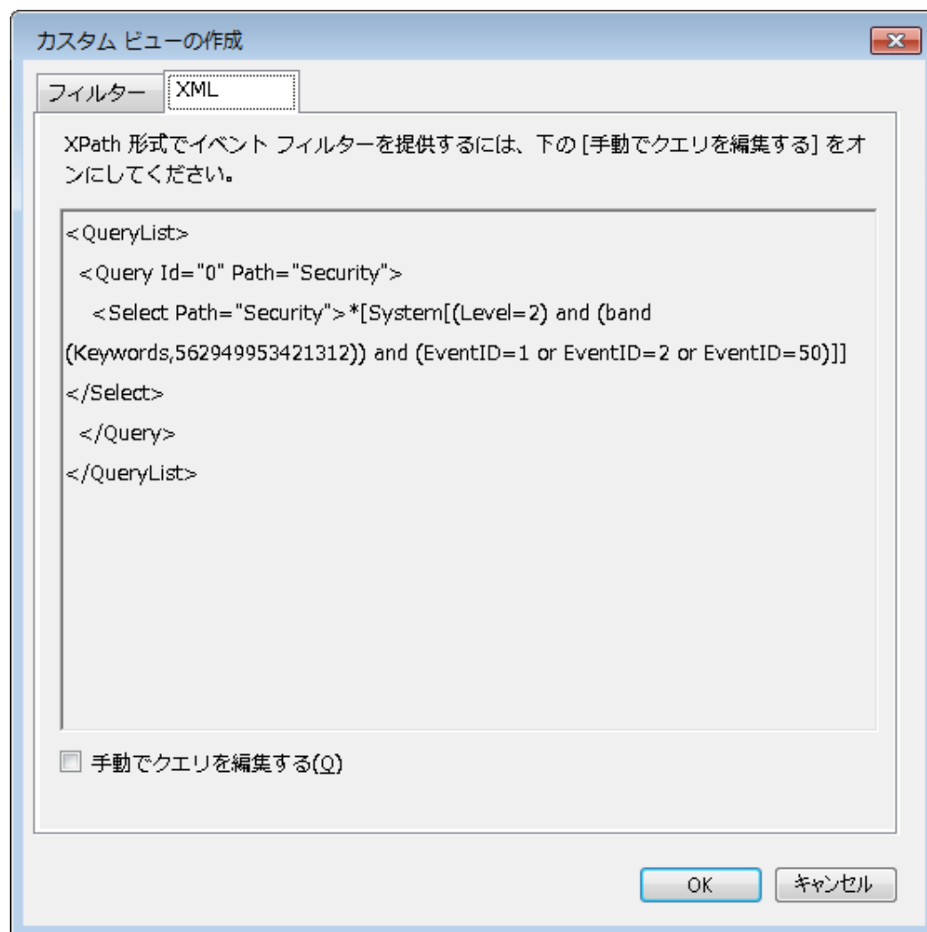
図 7-19 イベントビューア XMLタブ
