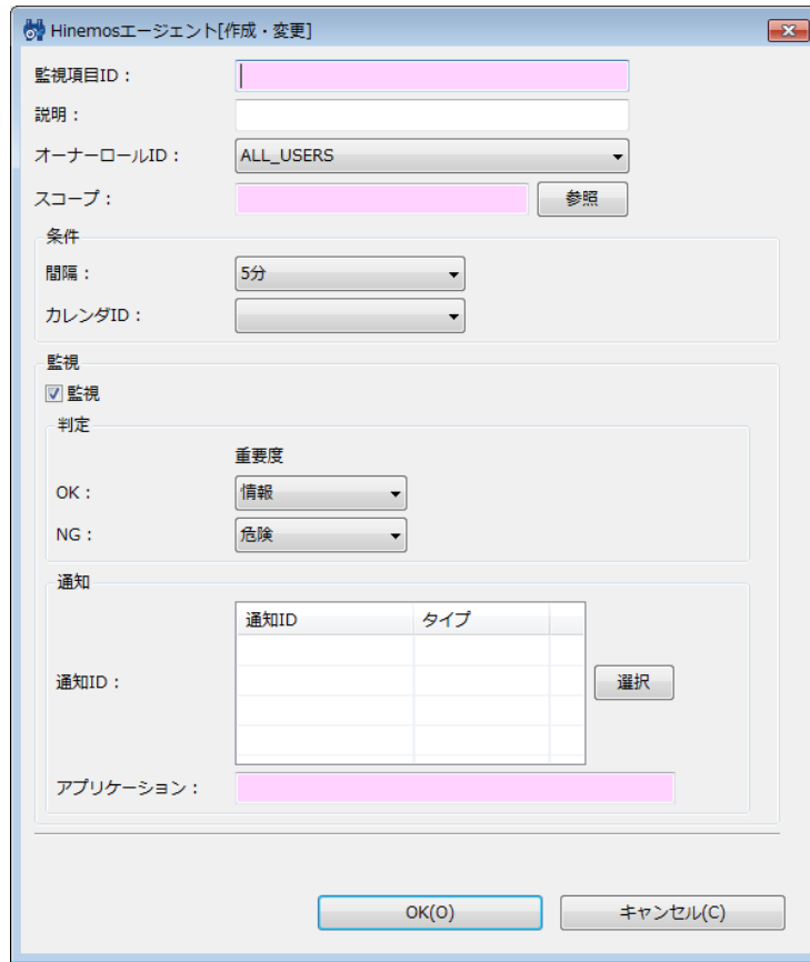
図 7-5 Hinemosエージェント[作成・変更]ダイアログ
